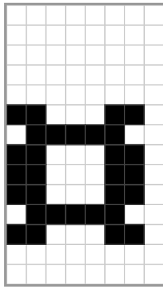
0x95
