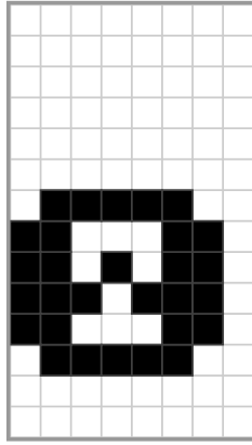
0x91
