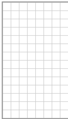
0x99
