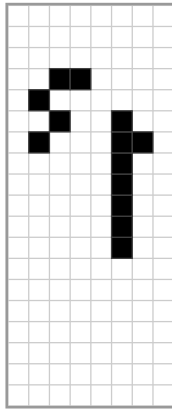
0x1D1
