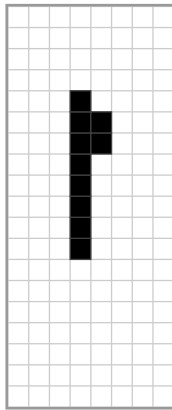
0x1D5
