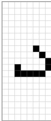
0x1DD
