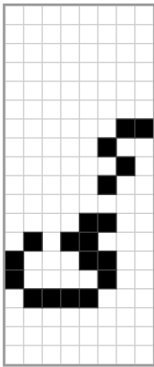
0x1D4
