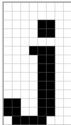
0x6A
